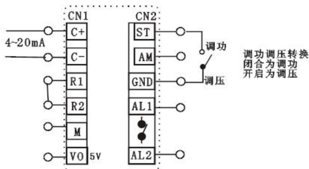
图 1-3: 全部功能实现接线及原理图
