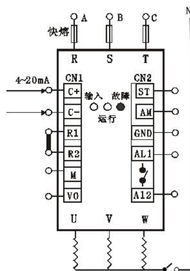
图 1-4: 自动运行接线方式
